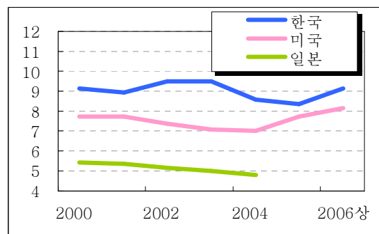
가계 지급이자/가처분소득
